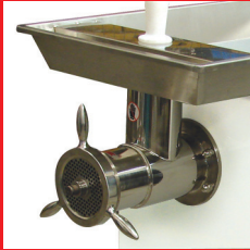
- Bandeja, cabezal, gusano y anillo de Acero Inoxidable
